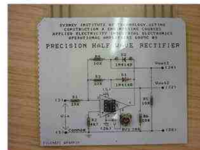
Page 229 Precision 1/2 wave rectifier
