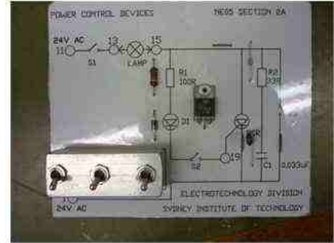
Page 147 SCR
