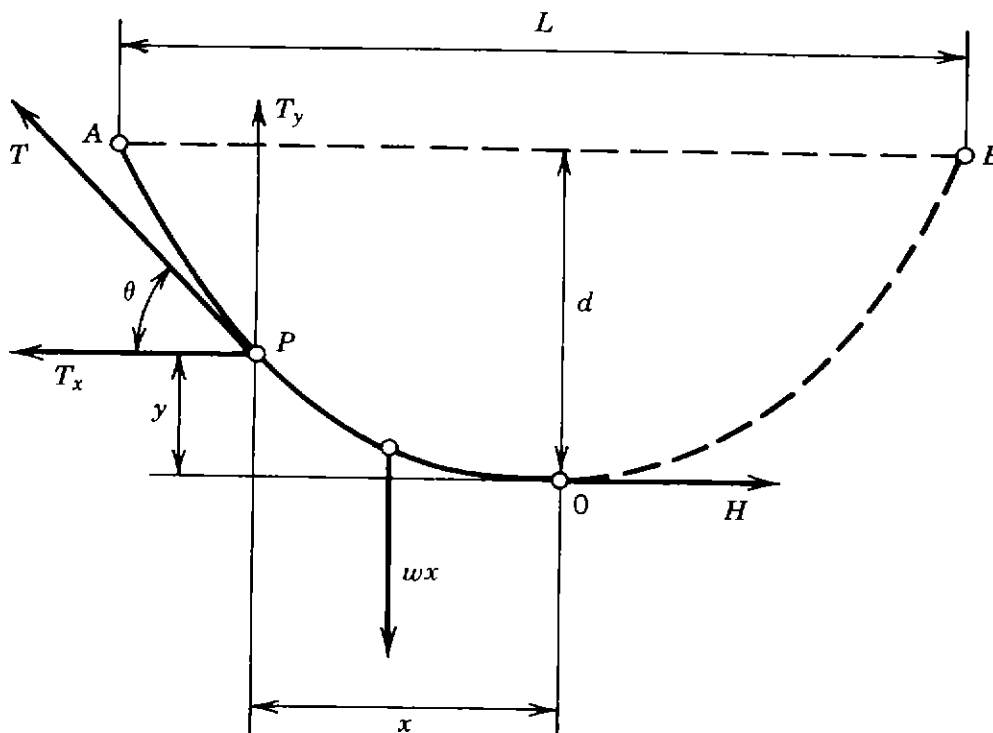
Figure 10.4. Parameters of parabola.
