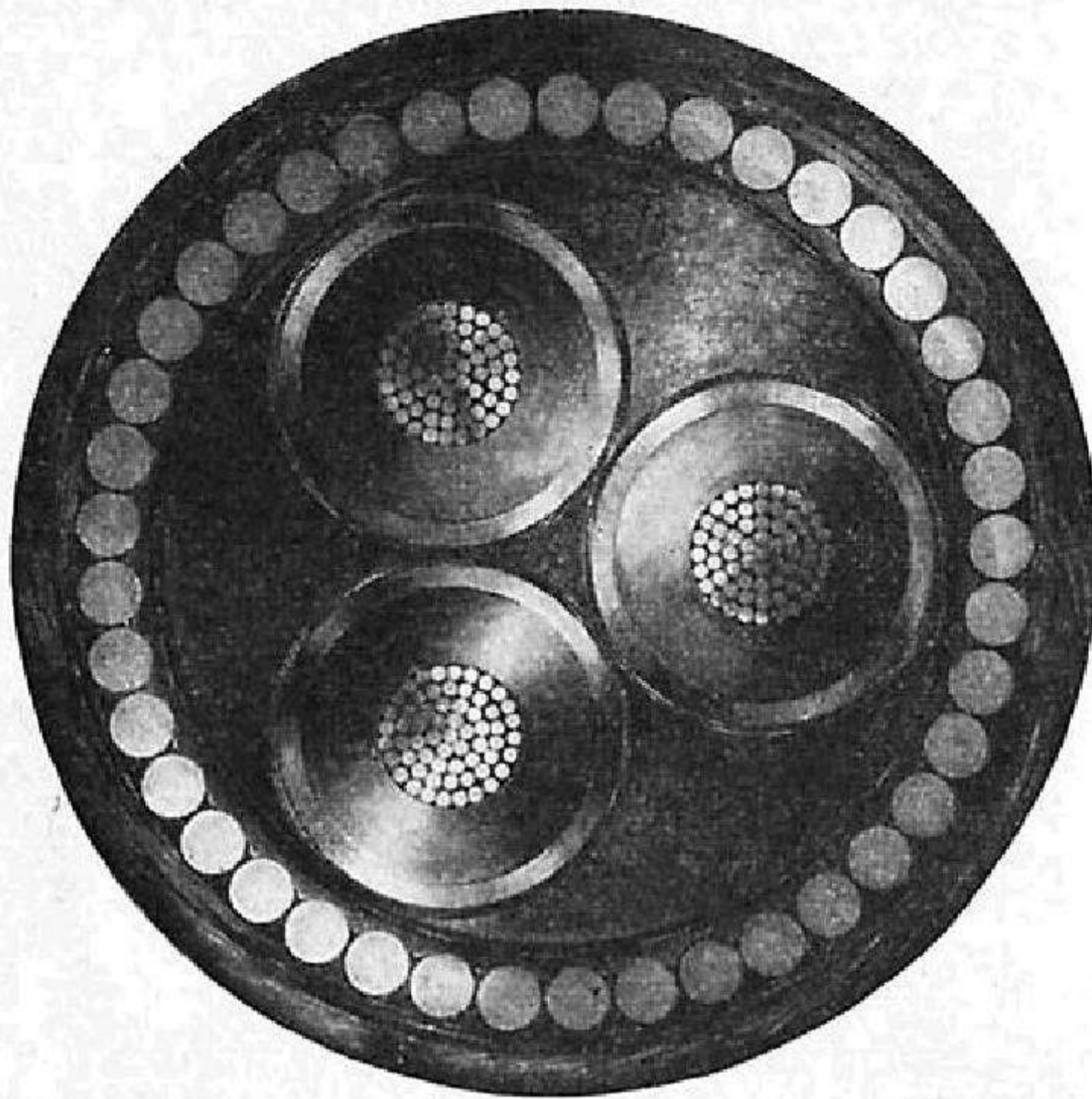
FIG. 72. "H.S.L."-TYPE CABLE (Siemens Bros.)
