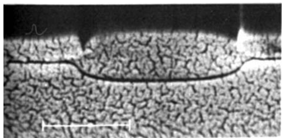
(C) LOPOS—2000Å Nitride/400Å Poly/300Å Oxide
