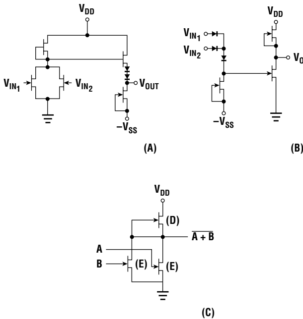
Figure 17.3 (A) Buffered FET logic (BFL). (B) Schottky diode FET logic (SDFL). (C) Direct coupled FET logic (DCFL).
