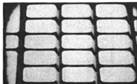
SEM TOP VIEW (100) DI ETCH
