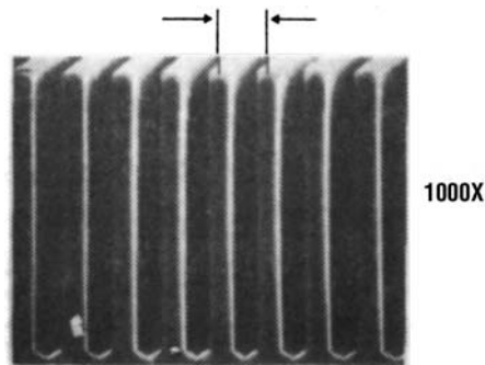
SEM CROSS-SECTIONAL VIEW (100) DI ETCH
